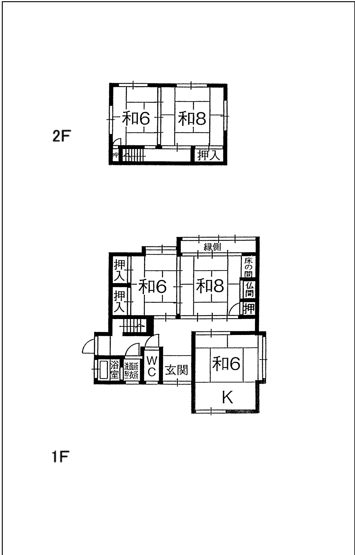
間取り図
