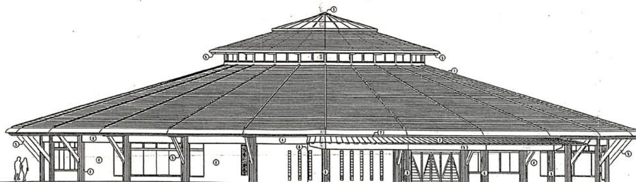
本館 西側立面図
