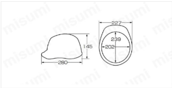
ヘルメットA-07WV型（通気孔付・雨垂れ防止溝付・衝撃吸収ライナー付）A-07WV-HA1E-K8-Aの寸法図
