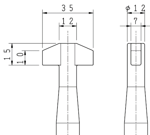
詳細 - B
