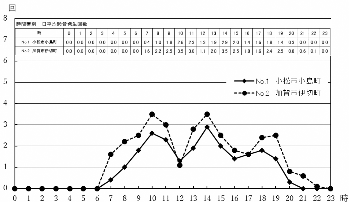
図－4 常時測定点における時間帯別一日平均騒音発生回数
