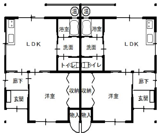
H17、18、19、20 木造 1LDK (81.62㎡)
