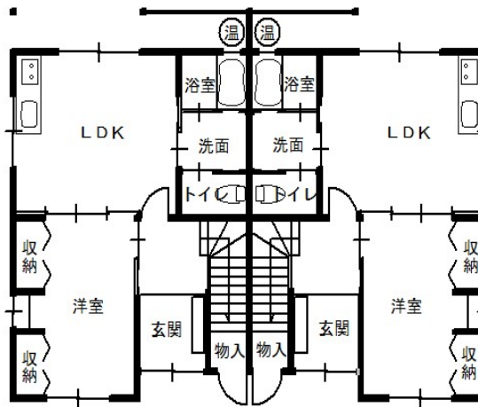
H17、18、19、20 木造 2LDK (125.04㎡)
