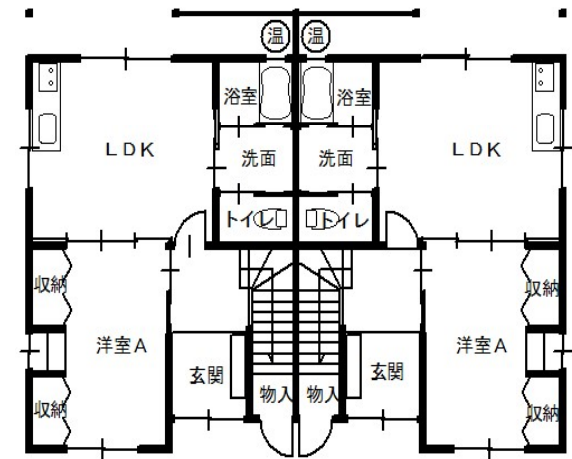
H17 木造 3LDK (147.07㎡)
