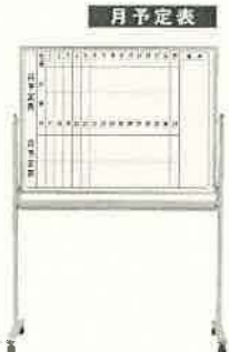
MH34TDMN ¥71,300 外形寸法 / W1326×D610×H1840 板面寸法 / W1210×H910 有効寸法 / W1170×H870
