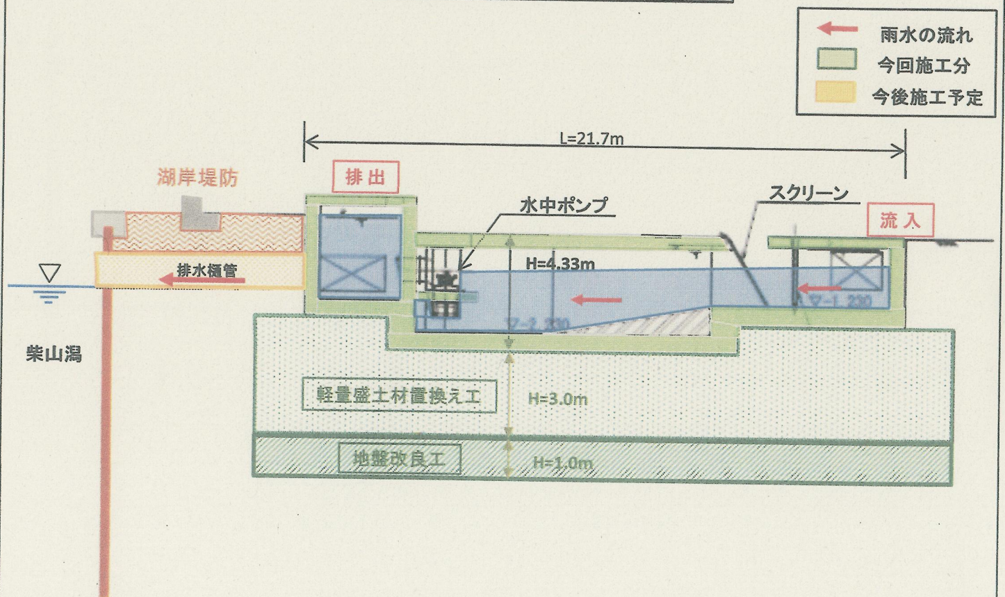
(仮称)湯の元公園ポンプ場断面図
