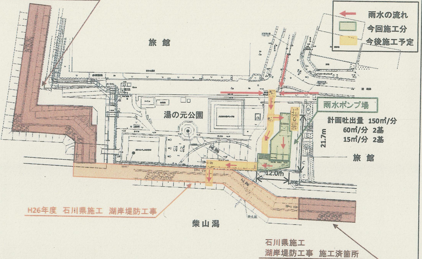
(仮称)湯の元公園ポンプ場位置図
