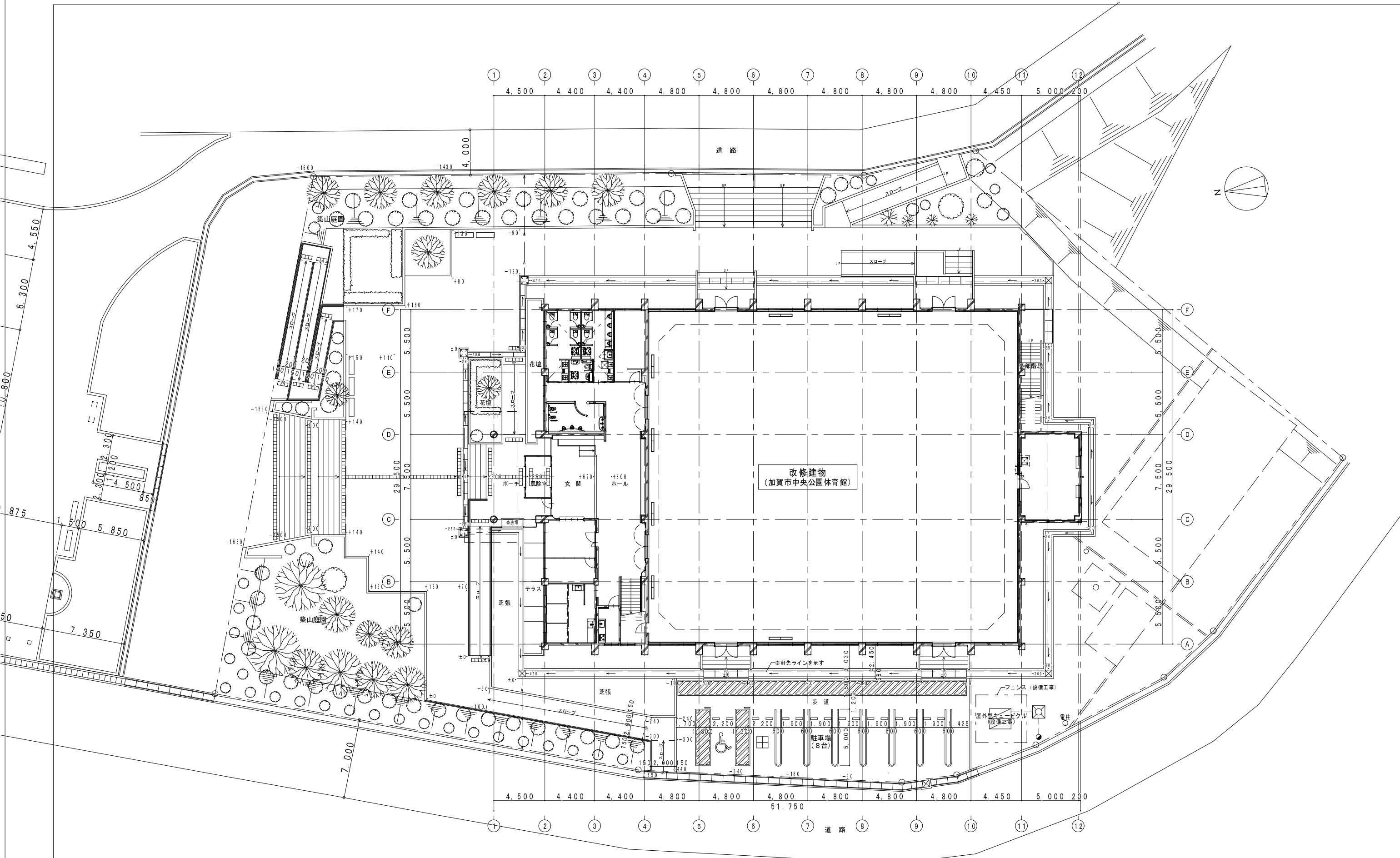
配置図
