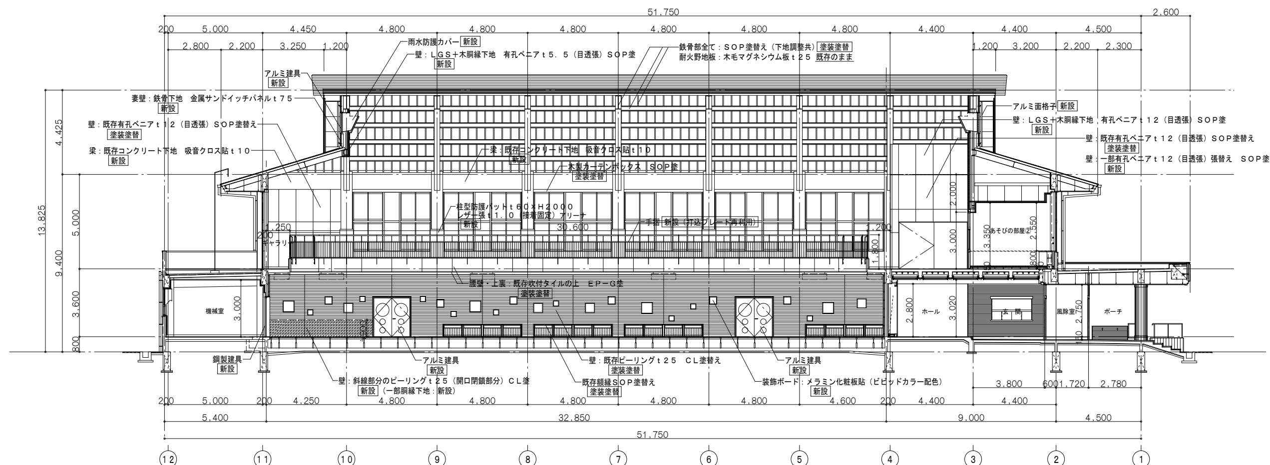
B-B 断面図
