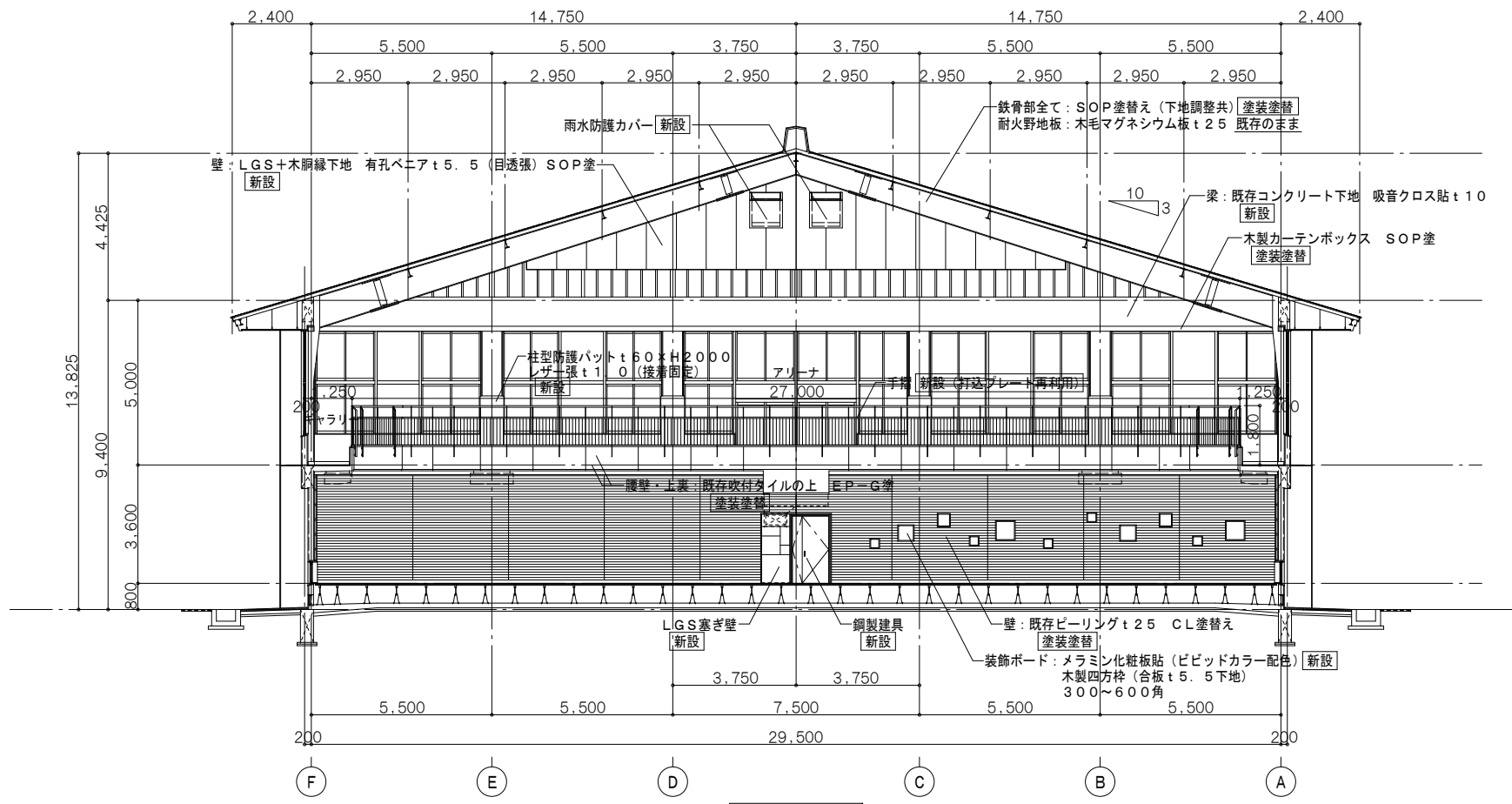
A-A 断面図
