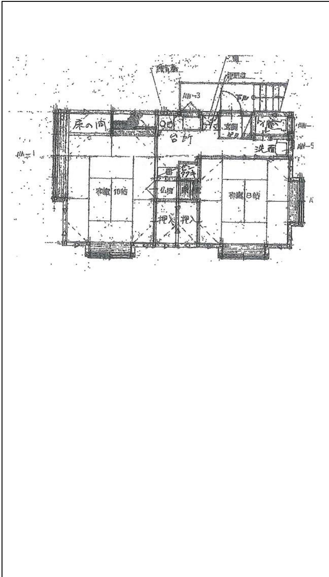
間取り図
